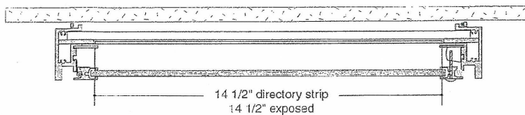
4 Section Scale: 3" = 1'-0"
