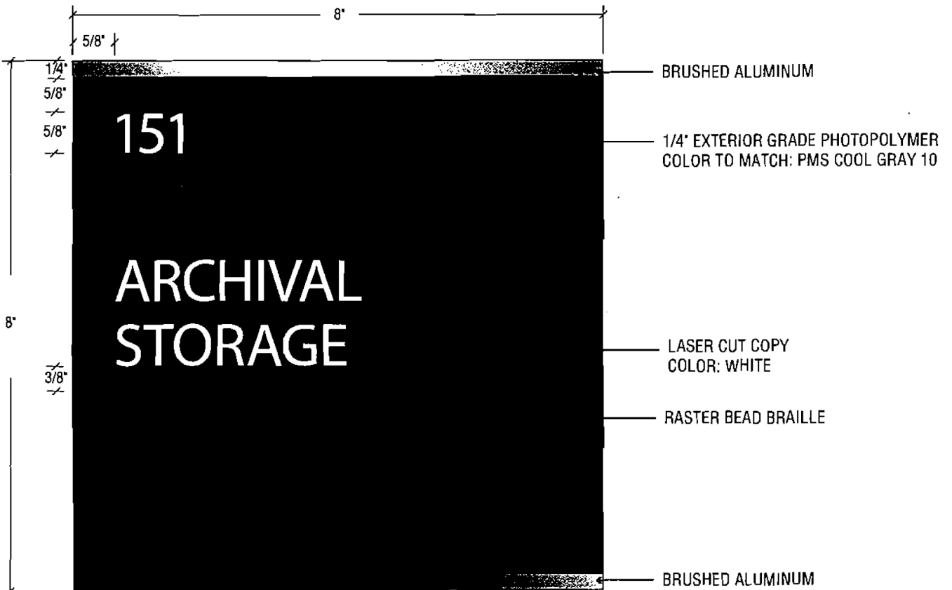
ELEVATION SCALE: 6" = 1'
