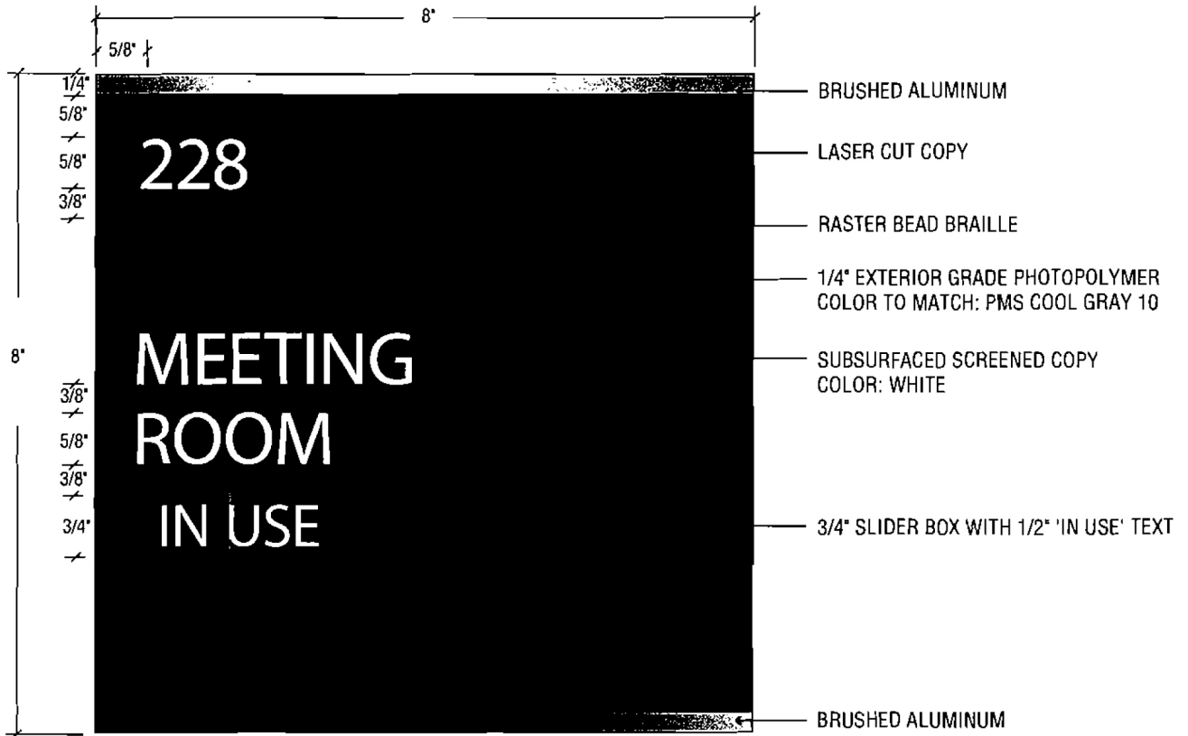
ELEVATION SCALE: 6" = 1'
