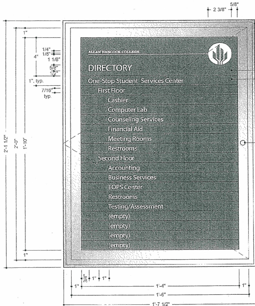
1 Front Scale: 3" = 1'-0"
